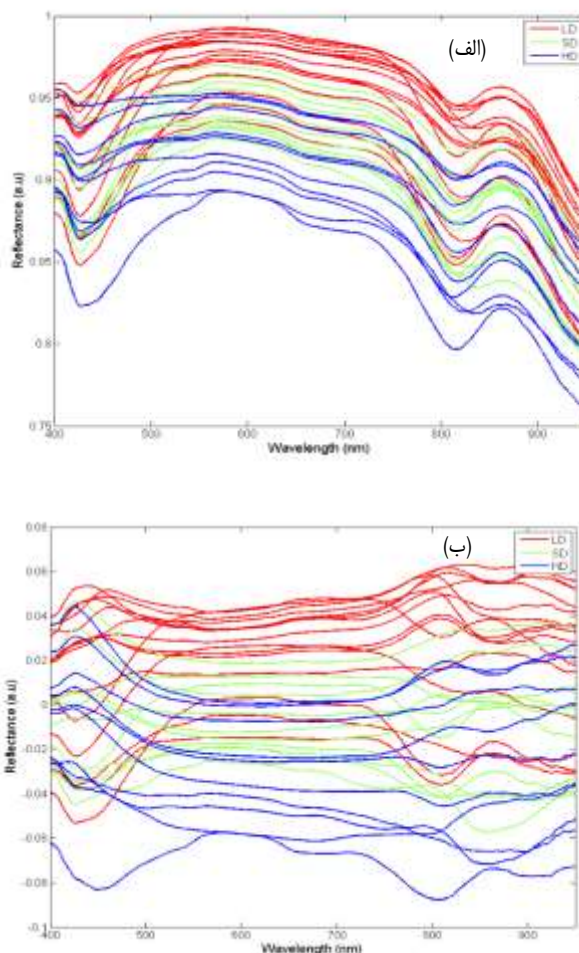
شکل ۴. الف) میانگین طیفی ۳۶ نمونه کالیبراسیون حاصل از تصویر برداری ابر طیفی با پیش‌پردازش هموارسازی ب) با پیش‌پردازش هموارسازی و مرکزسازی نسبت به میانگین.
