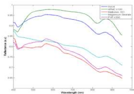
شکل ۳. میانگین طیفی مواد خام مورد استفاده در ساخت نمونه‌ها حاصل از تصویربرداری ابرطیفی با پیش پردازش هموارسازی.
