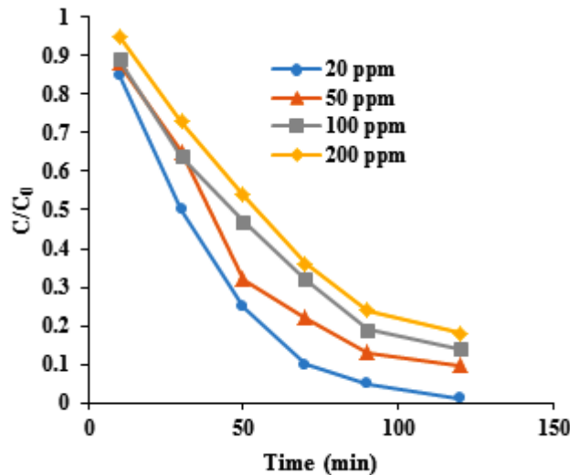
شکل ۶- اثر غلظت اولیه بر روی تخریب فوتوکاتالیستی رنگ اریوکروم بلک T.
