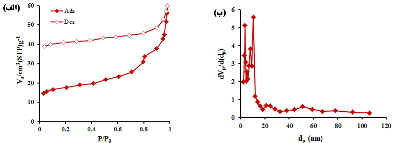
شکل ۳- ایزوترم جذب و واجذب گاز نیتروژن (الف) و نمودار توزیع اندازه حفره (BJH) (ب) مربوط به TMU-16.
