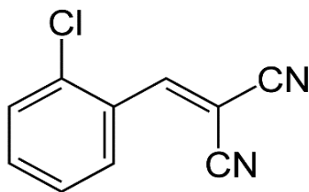
شکل ۱- ساختار شیمیایی ترکیب سیانو کربنی OCMB
