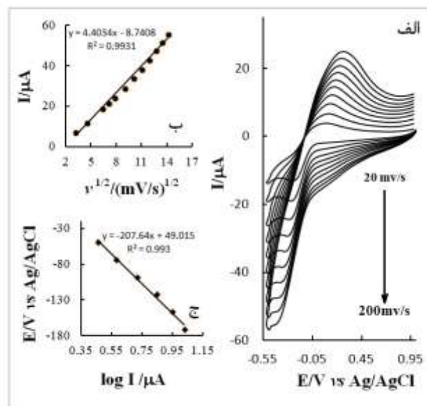
شکل ۴- (الف) ولتامتری چرخه‌ای الکتروکد خیمیر گرافن در سرعت روبش‌های مختلف در محلول ۰/۱ مولار بوریک اسید (pH=۳) حاوی ۱ mM اورانیل. سرعت‌های روبش ۲۰، ۴۰، ۶۰، ۸۰، ۱۰۰، ۱۲۰، ۱۴۰، ۱۶۰، ۱۸۰ و ۲۰۰ mV/s، (ب) تغییرات جریان پیک احیای اورانیل با ریشه دوم سرعت اسکن (د) نمودار تافل مربوط به ولتاموگرام در سرعت اسکن ۲۰ mV/s
