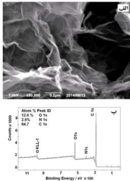
شکل ۳-۱- تصویر SEM گرافن اکسید احیاء شده (ب) طیف فوتوالکترون اشعه ی
