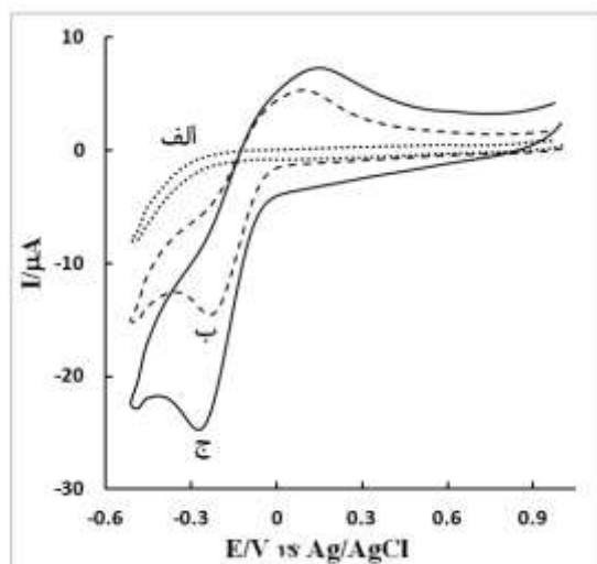
شکل ۲- ولتاموگرام‌های به‌دست‌آمده الف) در غیاب و ب و ج) به ترتیب در سطح الکتروود خمیر کربن و الکتروود خمیر گرافن در حضور محلول ۱ mM اورانیل در محلول بوریک اسید ۰/۱ مولار با \text{pH}=3 ، سرعت اسکن ۵۰ میلی ولت بر ثانیه
