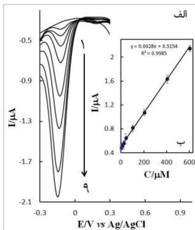
شکل ۵- الف) ولتاموگرامهای پالس تفاضلی محلول زمینه (۱) و محلول‌های (۲ تا ۹) حاوی غلظت‌های ۱، ۲، ۴، ۱۰، ۲۰، ۴۰، ۶۰، ۱۰۰، ۲۰۰، ۴۰۰، ۶۰۰ میکرومولار اورانیل در محلول بوریک اسید با pH=۳، (ب) نمودار جریان پیک بر حسب غلظت اورانیل
