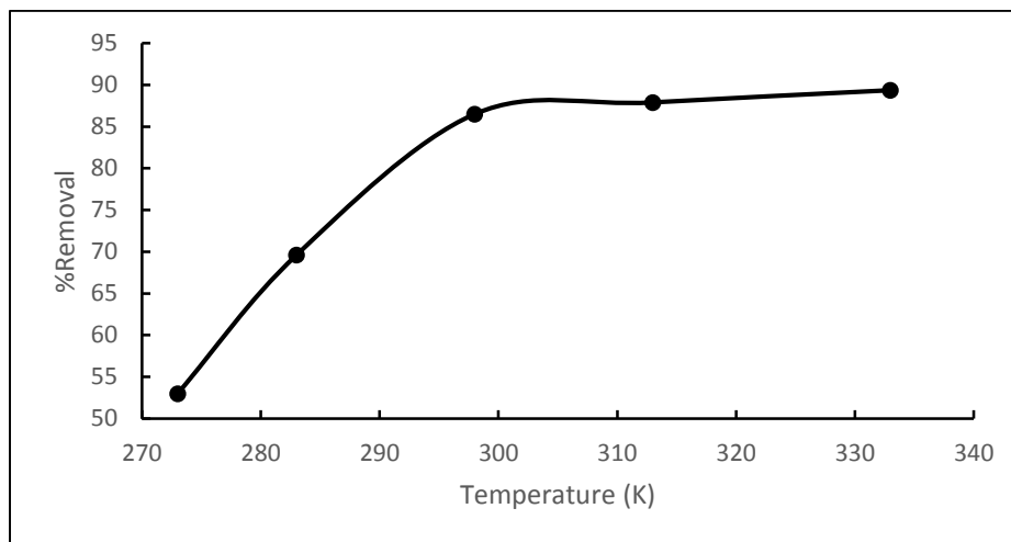
شکل ۸: اثر دما بر میزان جذب متیلن بلو توسط خاکستر گیاه کاکوتی
