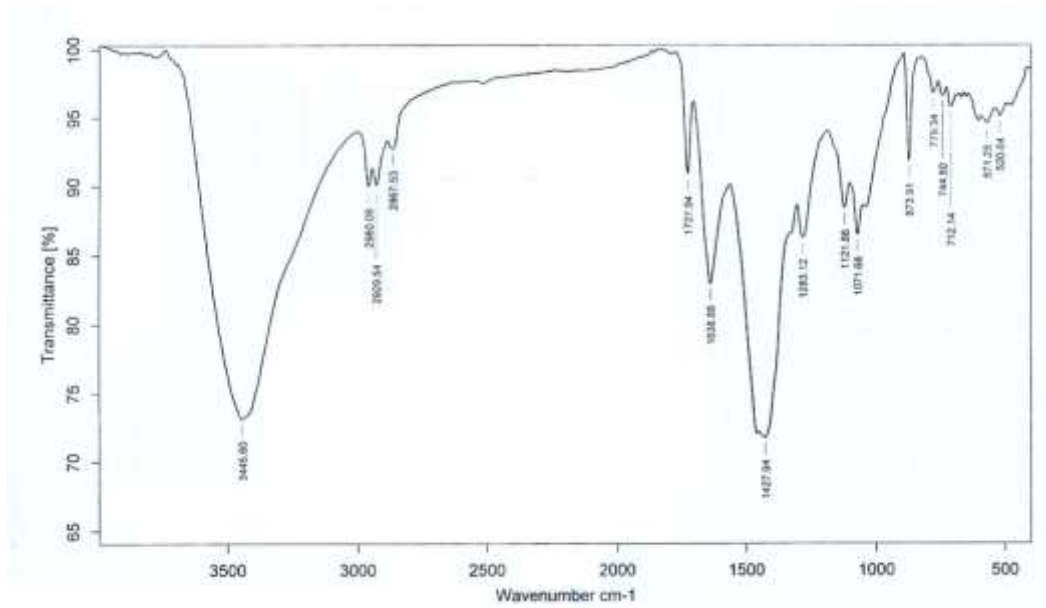
شکل ۱: طیف FT-IR خاکستر گیاه کاکوتی
