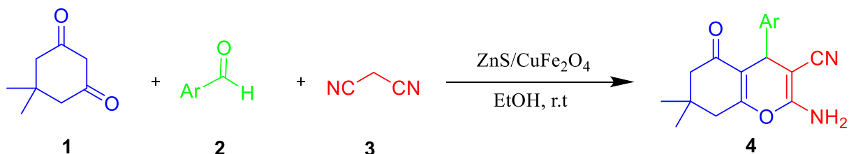
شکل ۱- واکنش کلی سنتز مشتقات ۲-آمینو-۳-سیانو-۴H-پیران
