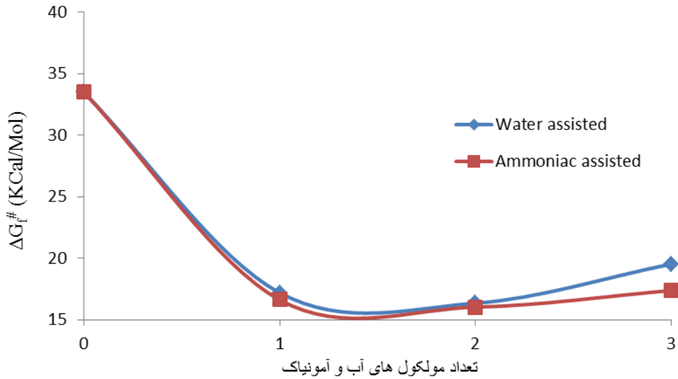
نمودار ۱- سد انرژی فعالسازی برای مسیر رفت در فاز گاز.
