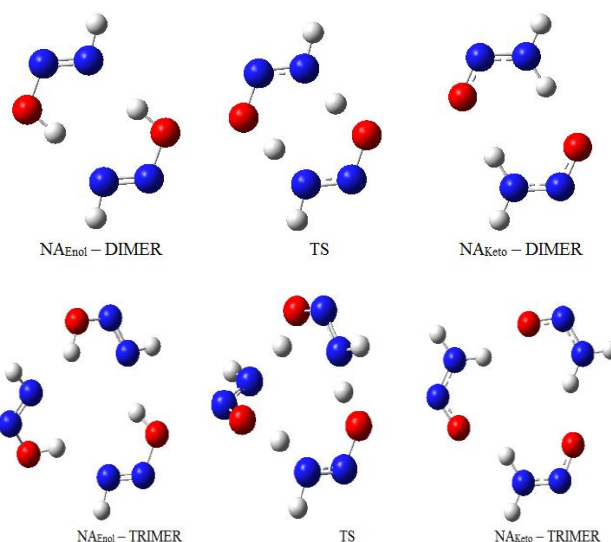
شکل-۳- توتومری نیتروز آمین به صورت دایمر و تریمر
