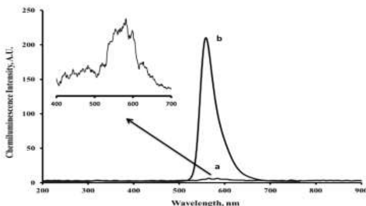
شکل ۹. a: طیف نورتایی شیمیایی محلول \text{Rdamim } 6G و b: طیف فلوئورسانس محلول \text{Rdamim } 6G
