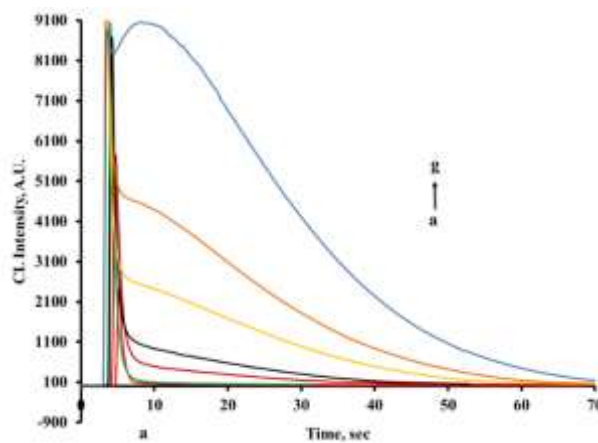
شکل ۲. نمودار پروفایل زمانی ترکیب پتیدین هیدروکلراید، به ترتیب از a تا g: شاهد، غلظت ۷ \times 10^{-7} ، ۵/۶ \times 10^{-۶} ، ۵/۶ \times 10^{-۵} ، ۱/۴ \times 10^{-۴} ، ۲/۸ \times 10^{-۴} و ۷ \times 10^{-۴} میلی‌مولار
