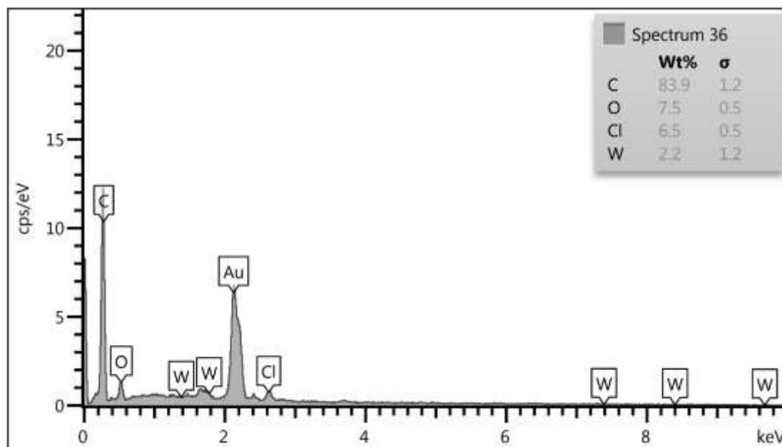
شکل ۵: طیف EDX فیلم متخلخل WO 3 /CNTs-Graphite-PVC
