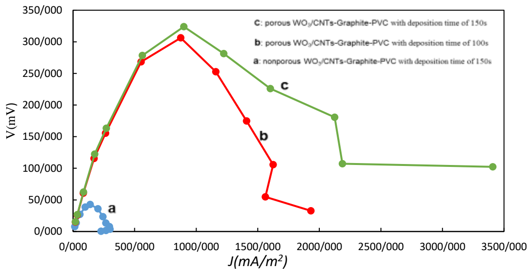
شکل ۶: نمودار تغییرات ولتاژ بر حسب چگالی جریان برای فیلم‌های ساخته شده
