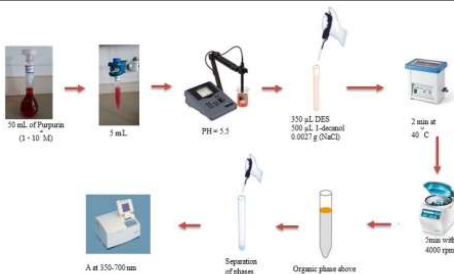
شکل ۱. شماتیک روش میکرواستخراج فاز مایع انجام شده برای پیش‌تخلیظ و اندازه‌گیری پورپورین.
