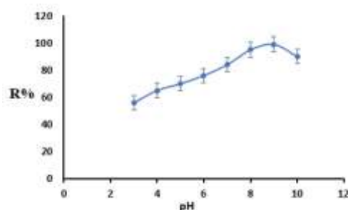
شکل ۴- اثر pH بر جذب جم فیبروزیل توسط نانو اکسید نیکل مغناطیسی
