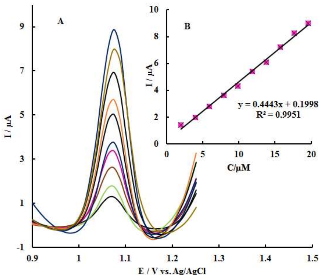
شکل ۷. (A) ولتاموگرام‌های پالس تفاضلی Nanoporous/GCE در غلظت های مختلف آسیکلوویر در گستره 1/99-19/6 \mu\text{M} در بافر فسفات با pH ۳ (دامنه پالس 50 mV، پهنای پالس 50 ms و سرعت روبش 20 mV/s). (B) نمودار I_p نسبت به غلظت آسیکلوویر
