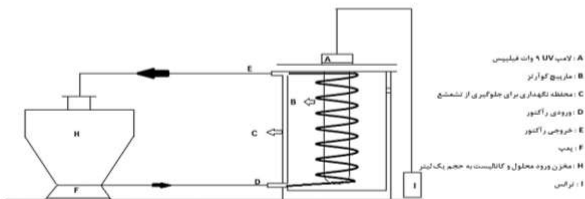
شکل ۱. شمای از راکتور فتوکاتالیستی لوله ای مارپیچ از جنس کوارتز به همراه تجهیزات جانبی مورد استفاده در کار حاضر.
