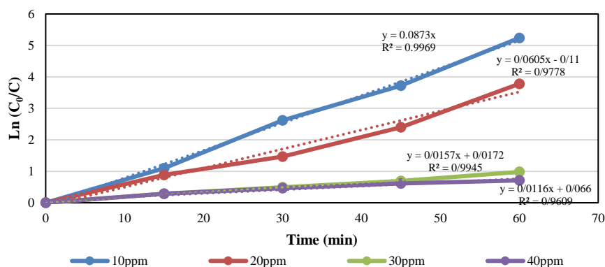
شکل ۱۱. بررسی سینتیک واکنش رنگبری فتوکاتالیست (ZnO-Ag-Zr)، مقدار کاتالیست ۳، ۱۰ و ۳۰ gr/lit، pH = ۱۰.
