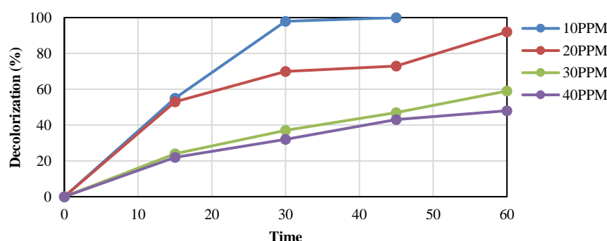
شکل ۱۰. تاثیر غلظت ابتدایی رنگ (RR198) بر راندمان رنگبری، مقدار فتوکاتالیست (ZnO-Ag-Zr) ۰,۳ g/l در pH=10، زمان ۶۰ دقیقه و غلظت رنگ ۲۰ ppm.
