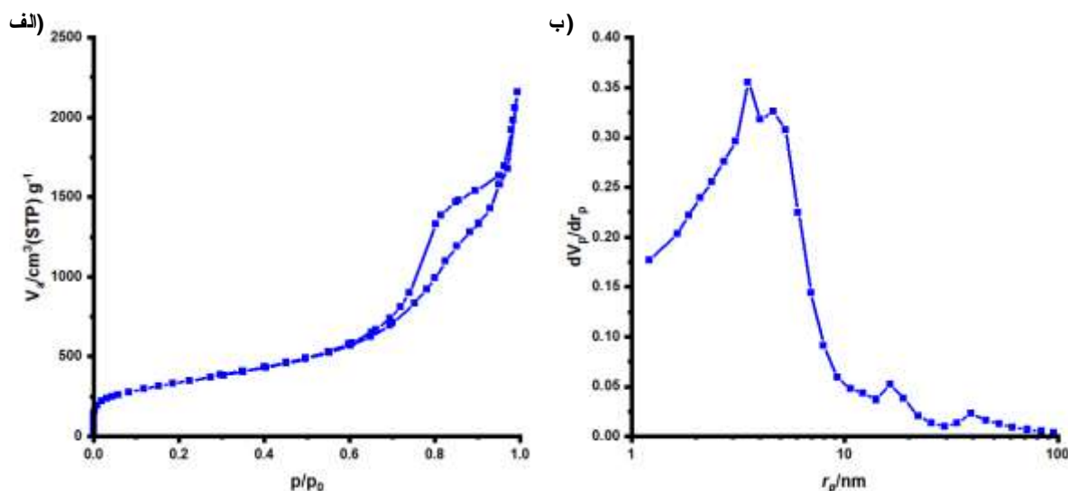
شکل ۸-الف) نمودار جذب و واجذب نیتروژن، ب) نمودار توزیع اندازه حفره‌ها ساختار N-CMS
