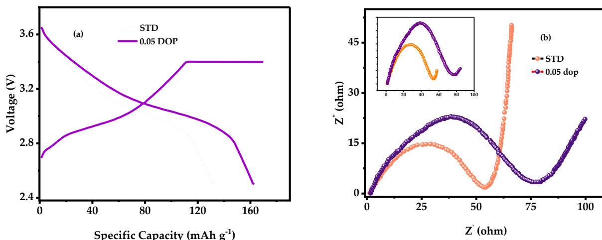
شکل ۶. الف) نمودار شارژ و دشارژ در باتری عاری و حاوی دوپامین (۰,۰۵ درصد وزنی) و ب) مقایسه مقاومت باتری با بهبود الکترولیت در دوپامین بهینه (۰,۰۵ درصد وزنی) بعد از ۲۰۰ چرخه
