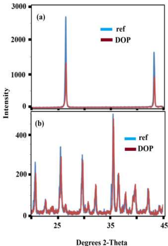
شکل ۹. نمودار XRD برای (الف) آند گرافیت و (ب) کاتد LFP، به ترتیب برای نمونه عاری از دوپامین (STD) و نمونه حاوی دوپامین بهینه (۰،۰۵ درصد وزنی)
