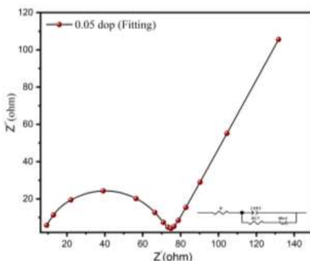
شکل ۷. الف) نمودار تطبیق (فیت کردن) مقاومت باتری با بهبود الکترولیت در دوپامین بهینه (۰,۰۵ درصد وزنی)
