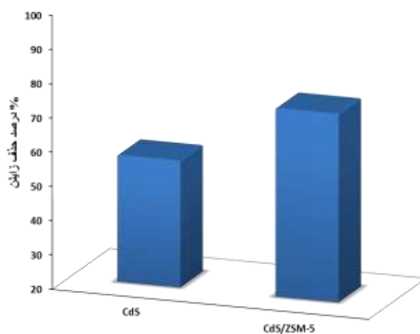
شکل ۵. درصد حذف بخارات زاینلین توسط CdS و CdS/ZSM-5 تثبیت شده روی لام های شیشه ای تحت تشعشع نور فرابنفش (غلظت زاینلین: ۳۰۰ ppm، مقدار فوتوکاتالیست: ۰/۱ g، زمان تست: ۷ ساعت)
