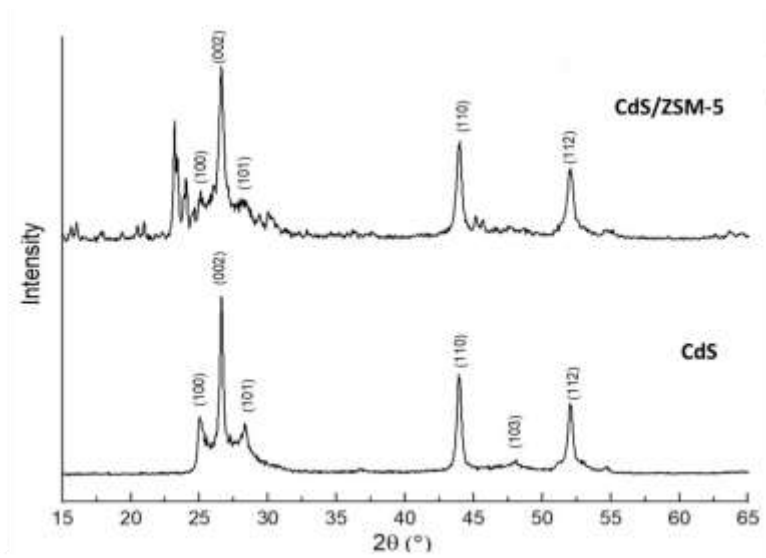
شکل ۲. الگوی پراش اشعه ایکس CdS/ZSM-5 و CdS
