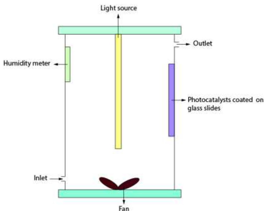
شکل ۱. شماتیک سامانه آزمایشگاهی استفاده شده برای تست فوتوتخریب بخارات زایلین
