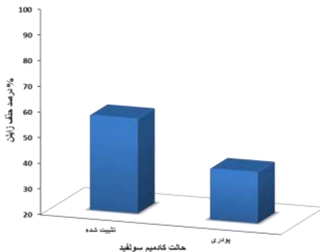
شکل ۴- درصد حذف بخارات زاینلین توسط کادمیم سولفید تحت تشعشع نور فرابنفش (غلظت زاینلین: ۳۰۰ ppm، مقدار فوتوکاتالیست: ۰/۱ g، زمان تست: ۷ ساعت)
