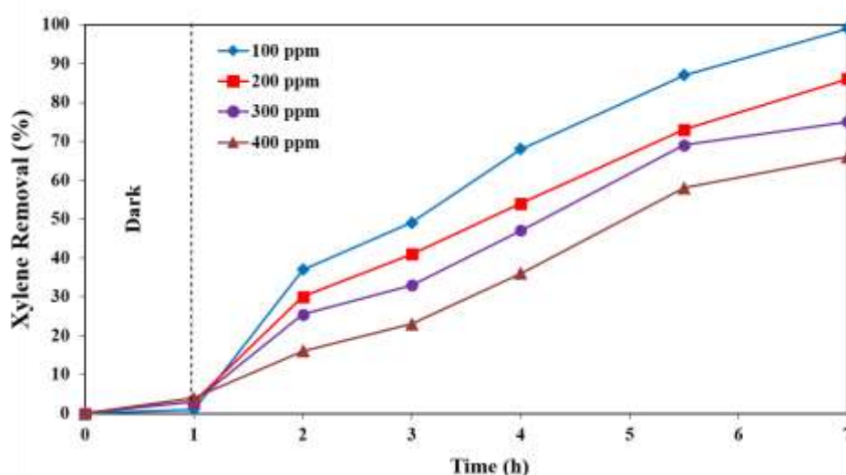
شکل ۶ درصد حذف بخارات زایلین با غلظت های مختلف توسط CdS/ZSM-5 تثبیت شده روی لام های شیشه ای تحت تشعشع نور فرابنفش (مقدار فوتوکاتالیست: ۰/۱ g و زمان تست: ۷ ساعت)
