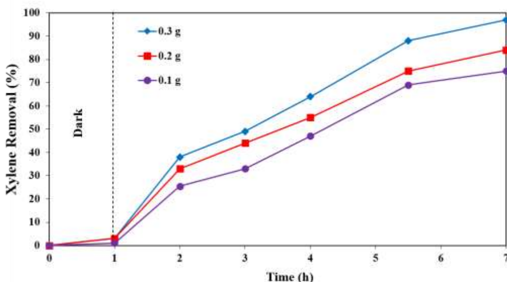
شکل ۷. درصد حذف بخارات زایلین توسط CdS/ZSM-5 با مقادیر مختلف تثبیت شده روی لام های شیشه ای تحت تشعشع نور فرابنفش (غلظت زایلین: ۳۰۰ ppm و زمان تست: ۷ ساعت)
