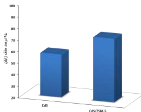
شکل ۵. درصد حذف بخارات زایلین توسط CdS و CdS/ZSM-5 تثبیت شده روی لام های شیشه ای تحت تشعشع نور فرابنفش (غلظت زایلین: ۳۰۰ ppm، مقدار فوتوکاتالیست: ۰/۱ g، زمان تست: ۷ ساعت)
