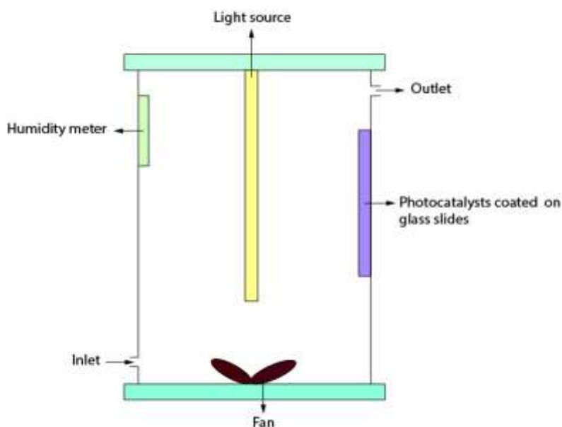
شکل ۱. شماتیک سامانه آزمایشگاهی استفاده شده برای تست فوتوتخریب بخارات زایلین
