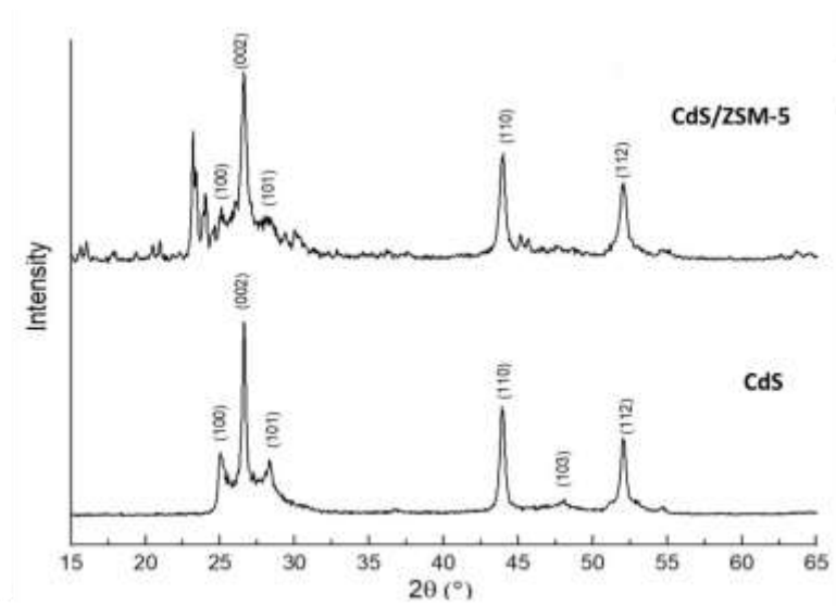
شکل ۲. الگوی پراش اشعه ایکس CdS و CdS/ZSM-5
