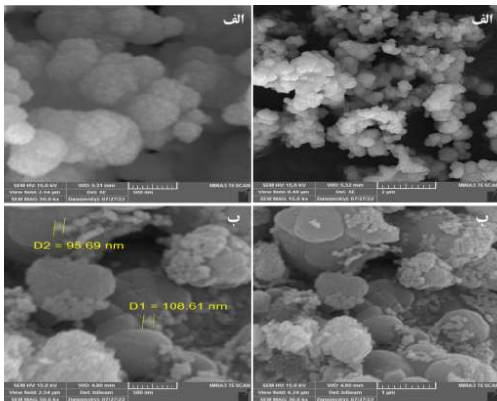
شکل ۳. تصاویر SEM (الف) CdS و (ب) CdS/ZSM-5
