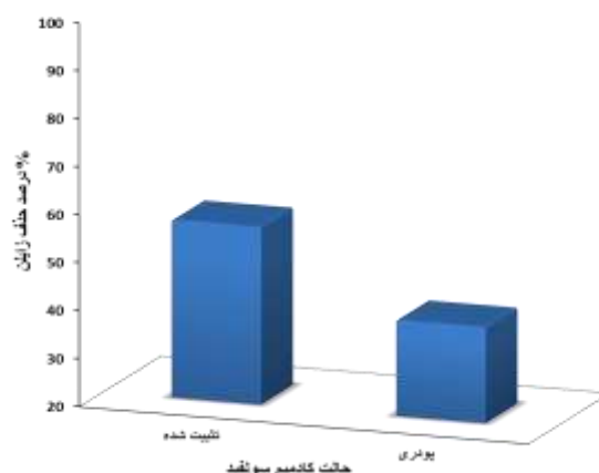
شکل ۴- درصد حذف بخارات زایلین توسط کادمیم سولفید تحت تشعشع نور فرابنفش (غلظت زایلین: ۳۰۰ ppm، مقدار فوتوکاتالیست: ۰/۱ g، زمان تست: ۷ ساعت)
