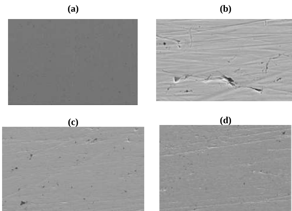
شکل ۴. تصاویر میکروسکوپ الکترونی روبشی مربوط به نمونه فولاد (a) ، نمونه فولاد در محیط خورنده بدون بازدارنده (b) ، نمونه فولاد در حضور بازدارنده SDS (c)، و نمونه فولاد در حضور بازدارنده DOTAB (d).
