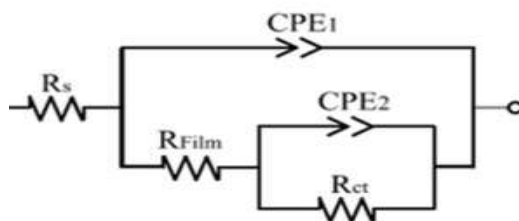
شکل ۳. مدار معادل مورد استفاده برای دیاگرام های نایکوئیست موجود در شکل ۲.
