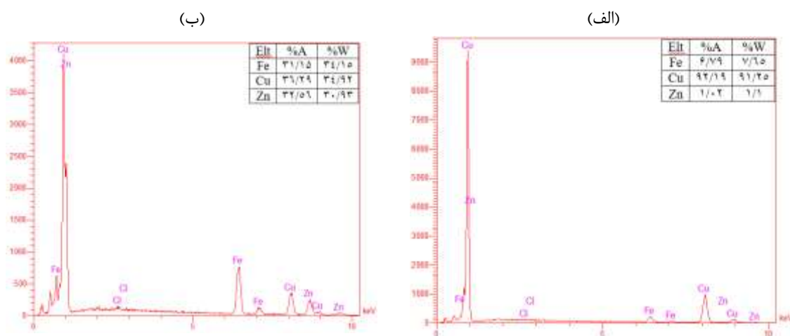
شکل ۳: آنالیز EDS نمونه لایه نشانی در نسبت مولی مس به روی (الف) ۱ به ۳ (ب) ۱ به ۱۰ (دما ۵۰ °C، زمان ۲۴۰ min، چگالی جریان (\frac{mA}{cm^2}) ۱)
