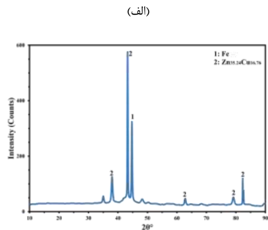
شکل ۱۰: (الف) الگوی پراش اشعه ایکس و (ب) تصویر میکروسکوپی الکترونی روبشی سطح مقطع نمونه لایه‌نشانی شده تحت شرایط نسبت مولی مس به روی ۱ به ۳، دمای 50^{\circ}\text{C} ، زمان ۲۴۰ min و چگالی جریان 5 \frac{\text{mA}}{\text{cm}^2}
