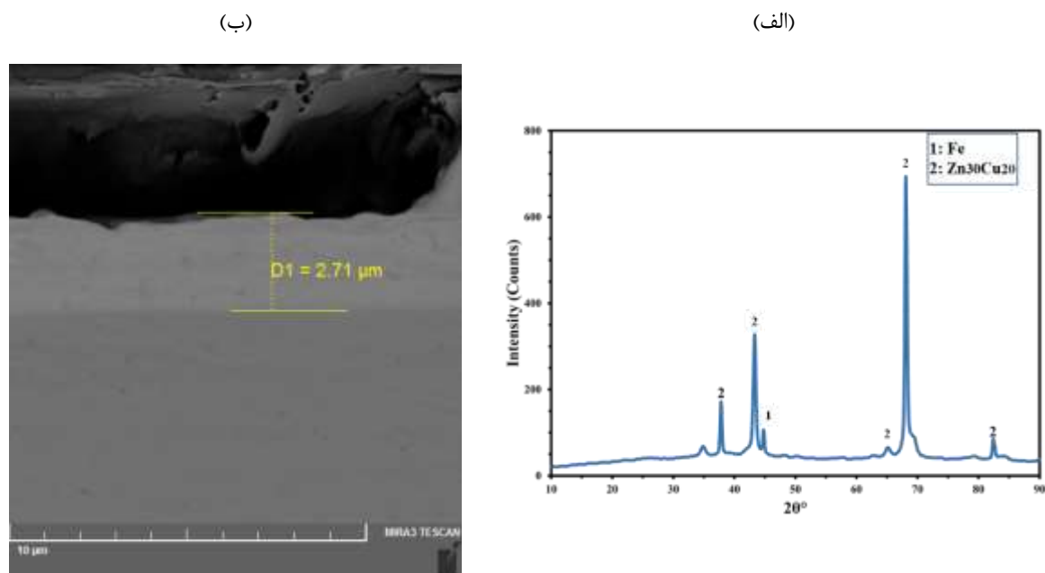
شکل ۱۴: (الف) الگوی پراش اشعه ایکس و (ب) تصویر میکروسکوپی الکترونی روبشی سطح مقطع نمونه لایه‌نشانی شده با نسبت مولی مس به روی ۱ به ۵ تحت شرایط دمای °C ۵۰، زمان ۲۴۰ min و چگالی جریان (\frac{mA}{cm^2}) ۵
