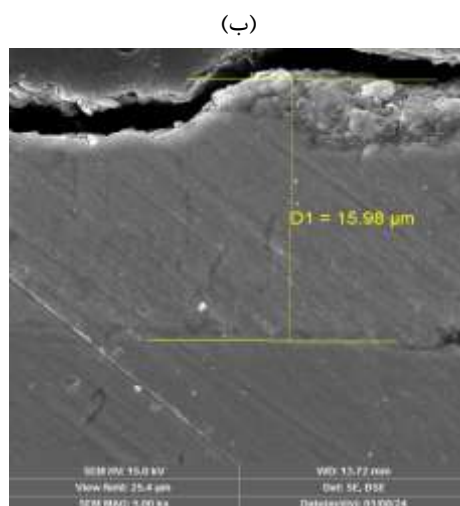
شکل ۱۰: (الف) الگوی پراش اشعه ایکس و (ب) تصویر میکروسکوپی الکترونی روبشی سطح مقطع نمونه لایه‌نشانی شده تحت شرایط نسبت مولی مس به روی ۱ به ۳، دمای 50^{\circ}\text{C} ، زمان ۲۴۰ min و چگالی جریان 5 \frac{\text{mA}}{\text{cm}^2}
